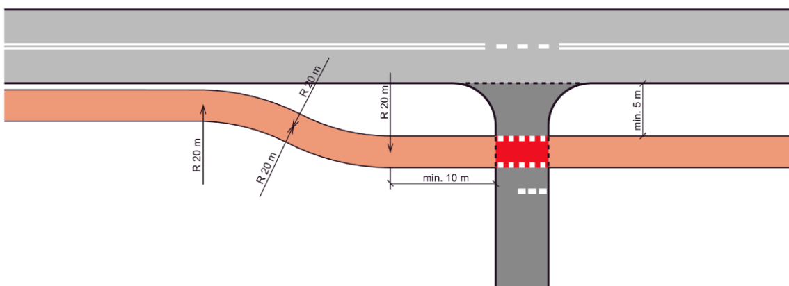
Rys.16 – Przekładnia drogi dla rowerów ze zjazdem publicznym
