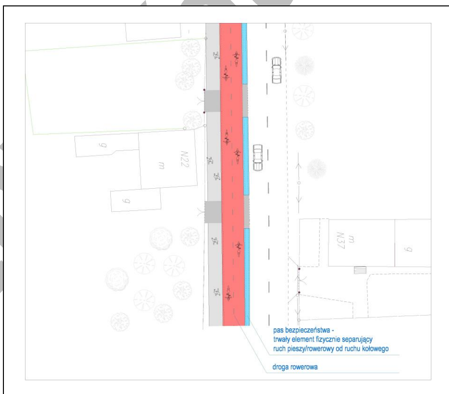
Rys. 10 – przykładowe rozwiązanie prowadzenia ruchu rowerowego i pieszego na odcinku przejścia przez małą miejscowość
