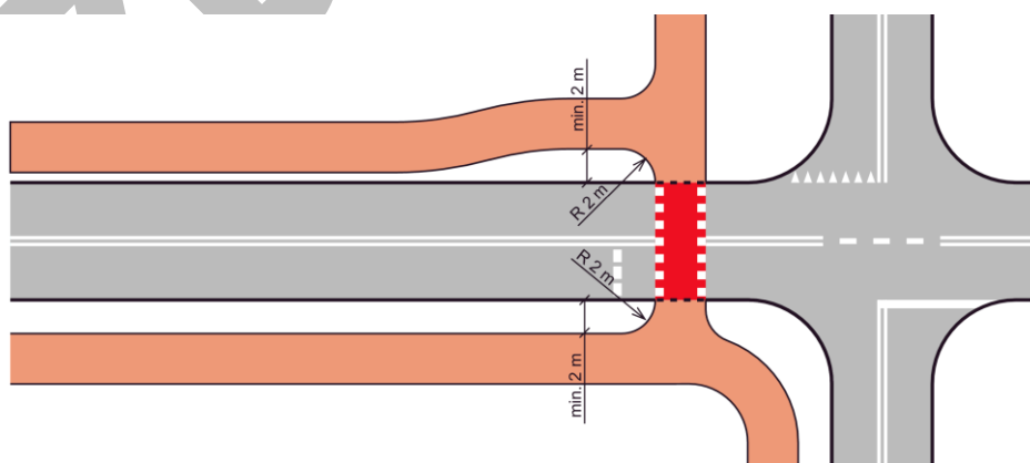
Rys. 19 – Przekięcie drogi dla rowerów ze wlotem skrzy¿owania posiadajãcym pierwszeństwo przejazdu
