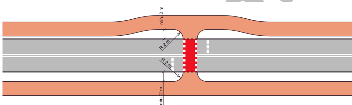
Rys. 20 – Przekucie drogi dla rowerów z drogą poza obrębem skrzyżowania
