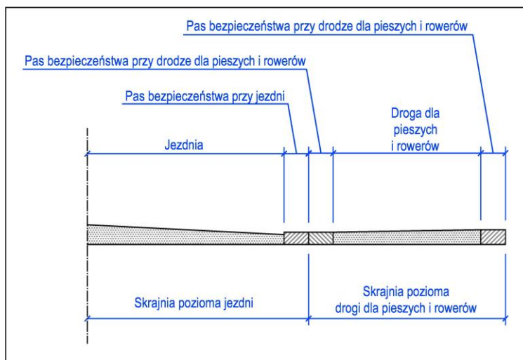
Rys. 3 – sąsiedowanie skrajni elementów infrastruktury drogowej
