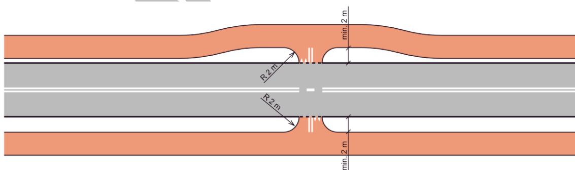
Rys. 21 – Przekucie drogi dla rowerów z drogą o dużym natężeniu ruchu pojazdów poza obrębem skrzyżowania
