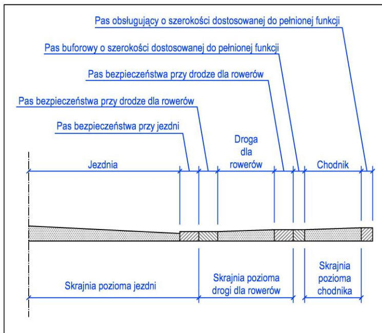
Rys. 2 – sąsiedowanie skrajni elementów infrastruktury drogowej
