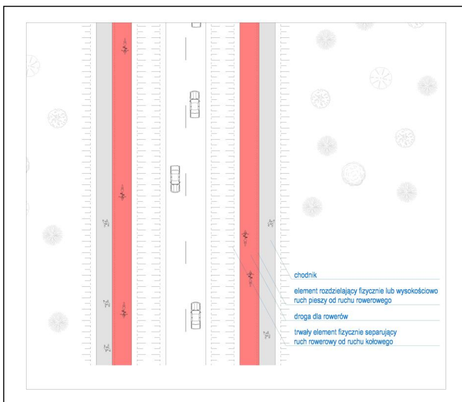
Rys. 8 – przykładowe rozwiązanie prowadzenia ruchu rowerowego i pieszego na odcinku drogi przebiegającym przez tereny niezurbanizowane
