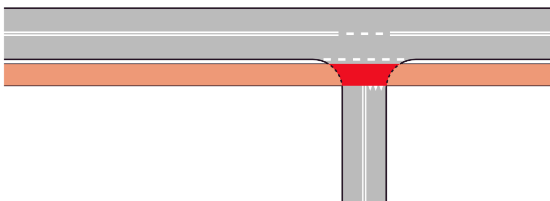
Rys. 18 – Przekięcie drogi dla rowerów ze wlotem podporzãdkowanym skrzy¿owania o małym natę¿eniu ruchu pojazdów
