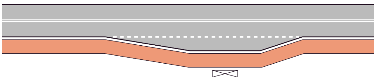
Rys. 25 – Prowadzenie drogi dla rowerów w obrębie przystanku komunikacji zbiorowej w przypadku małego natężenia ruchu pieszych
