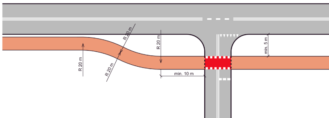
Rys. 17 – Przekięcie drogi dla rowerów ze wlotem podporzãdkowanym skrzy¿owania
